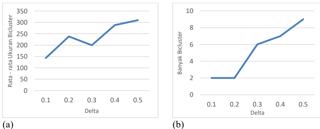
Gambar 2. (a) Grafik Perbandingan Rata – Rata Ukuran Bicluster vs Delta (b) Grafik Perbandingan Banyak Bicluster vs Delta
