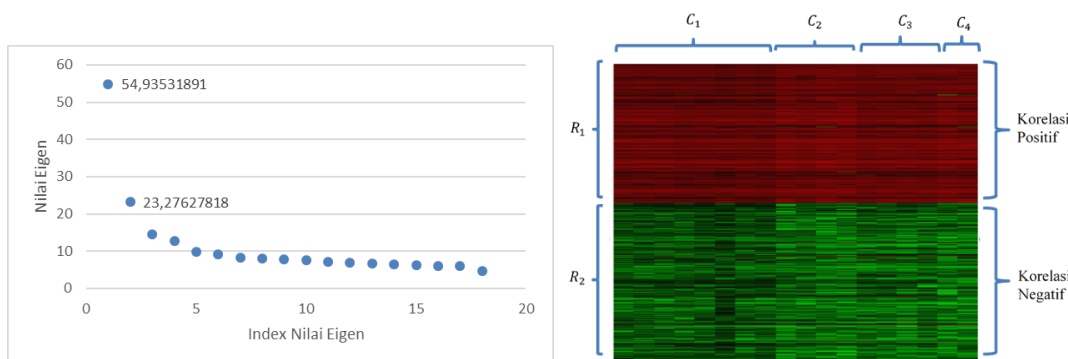
5(a) Grafik Penyebaran Nilai Eigen 5(b) Hasil Heatmap Dari Pembentukan Original Biclusters
