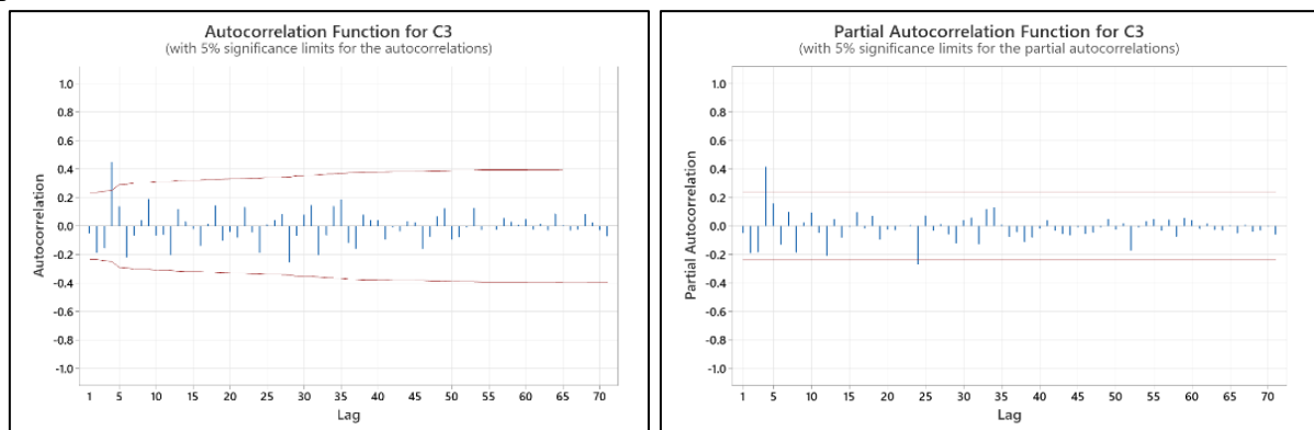
Gambar 3. Plot ACF dan PACF Data Produksi Padi
