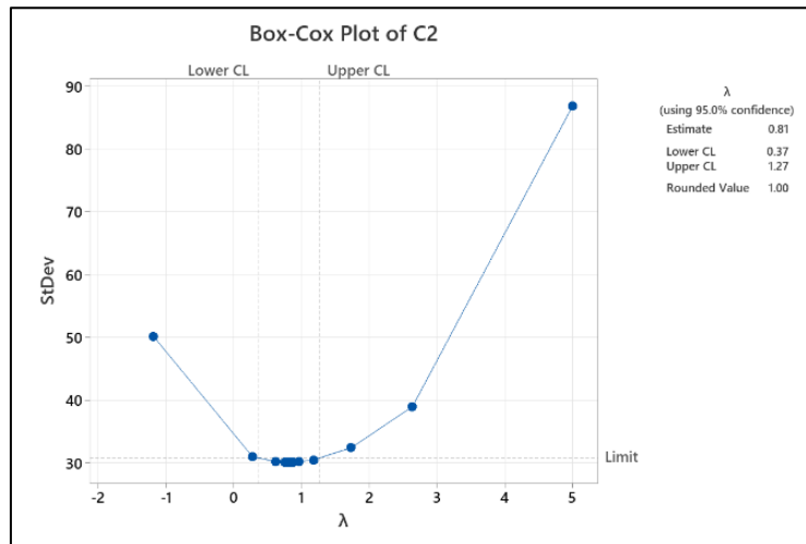
Gambar 2. Plot Box-Cox Produksi Padi di Kabupaten Buleleng
