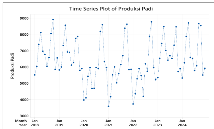
Gambar 1. Plot Data Produksi Padi
