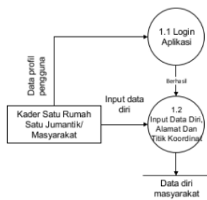
9 Gambar 5 Data Flow Diagram Level 2 Pendaftaran Pengguna
