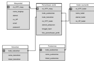
Gambar 8 Tabel Relasi Database
