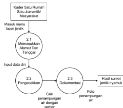
2 Gambar 6 Data Flow Diagram (DFD) level 2 Pemeriksaan Jentik Nyamuk
